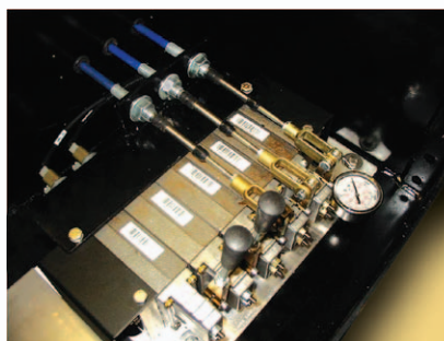
PVG 32 Manual Actuation
