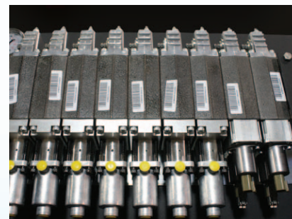
PVG 32 Air Actuation
